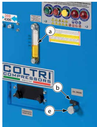
MCH-13-16/ET MINI SILENT EVO
